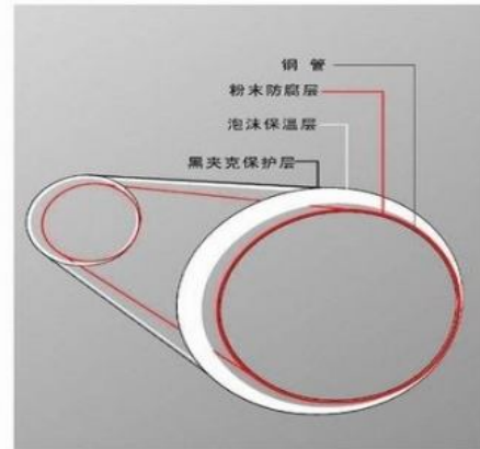
钢管道防腐保温“新一步法”粉末、泡沫黑夹克新结构
